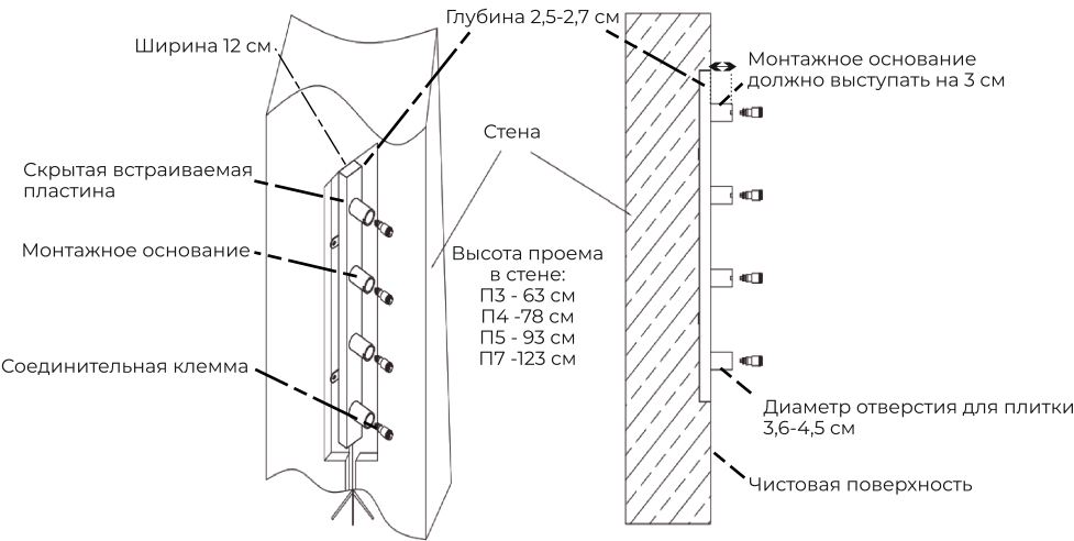
Схема 1. Подключение к электросети
