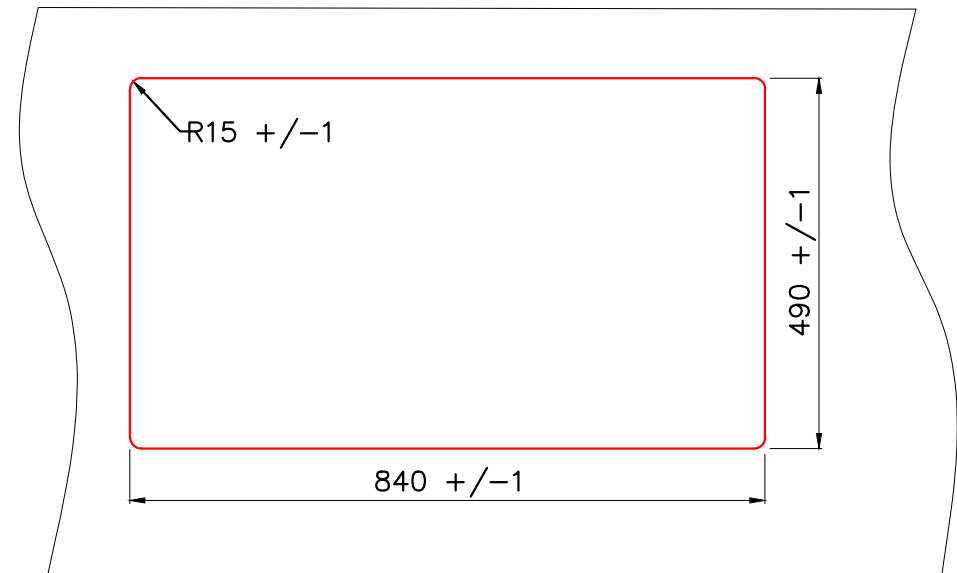
Врезной монтаж мойки (I)
